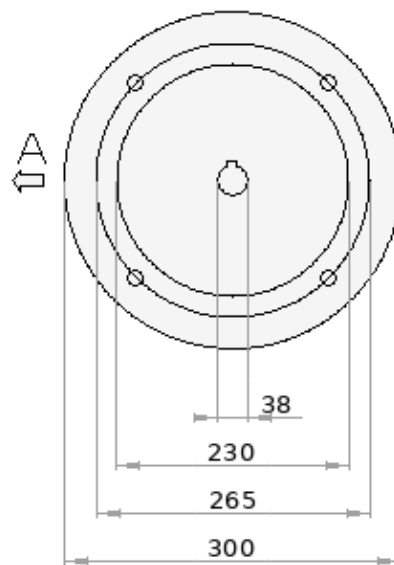
Flangia in ingresso, vista da A
